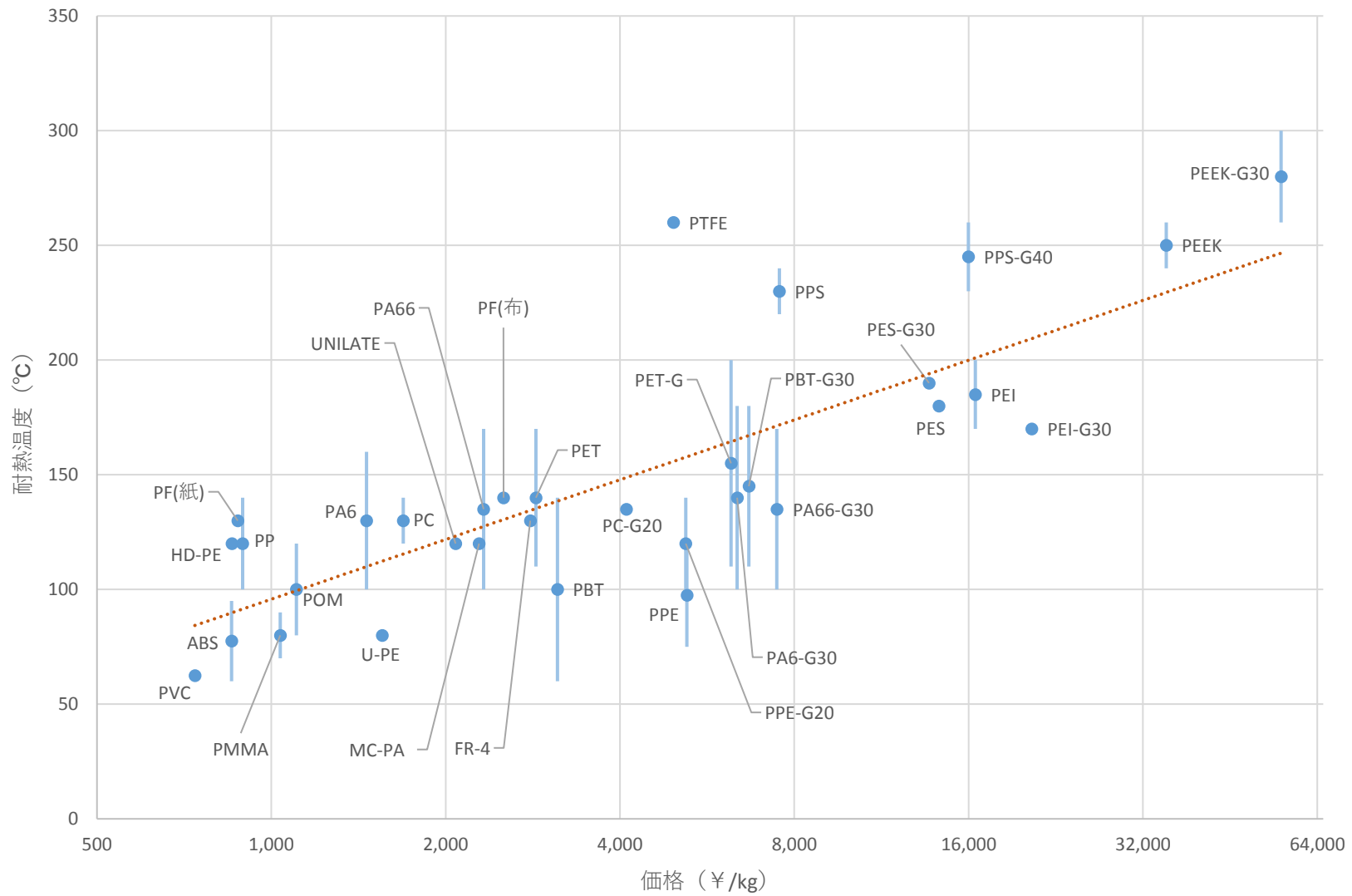
(樹脂) 価格と耐熱温度の関係
